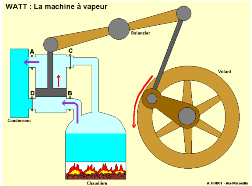
La machine à vapeur de James Watt
